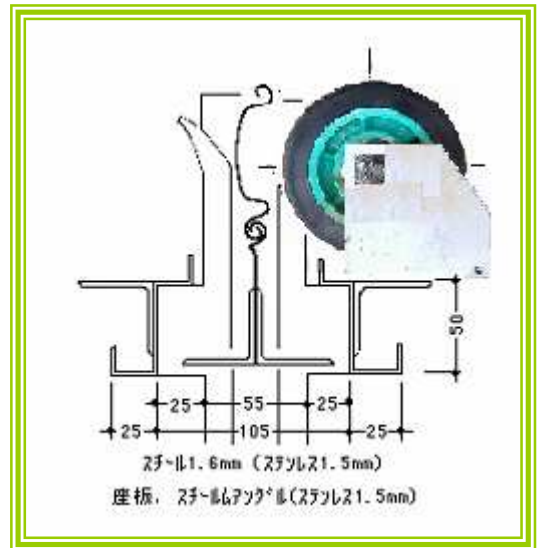
納まり図
